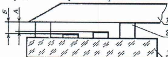
Рисунок 1 - Образец для определения значения просвета
